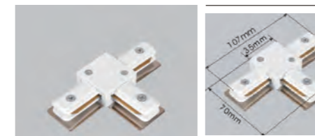
T-connector
