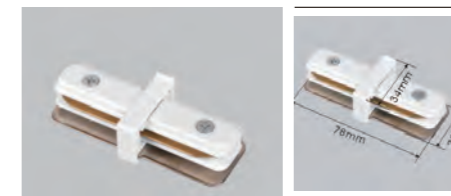
Straight connector MINI
